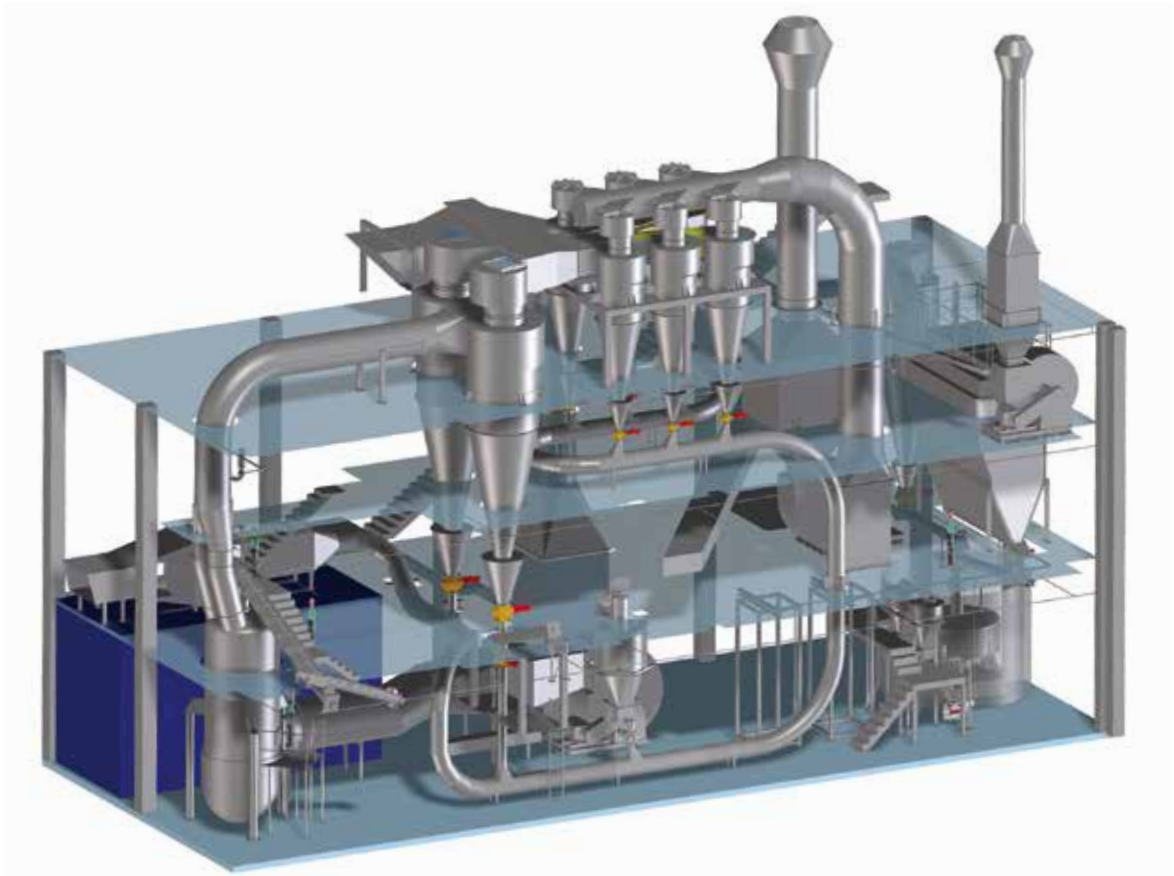
Beispiel einer Komplettanlage zur Stärketrocknung und -kühlung
